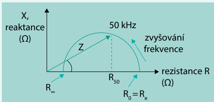
Schéma. Typický průběh bioimpedančního vektoru v komplexní rovině při frekvenci proměnné od nuly až po řádově MHz a schéma náhradního elektrického obvodu simulujícího impedanci živé tkáně
