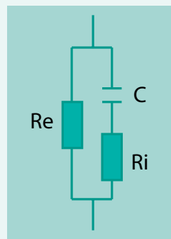
Schéma. Typický průběh bioimpedančního vektoru v komplexní rovině při frekvenci proměnné od nuly až po řádově MHz a schéma náhradního elektrického obvodu simulujícího impedanci živé tkáně
